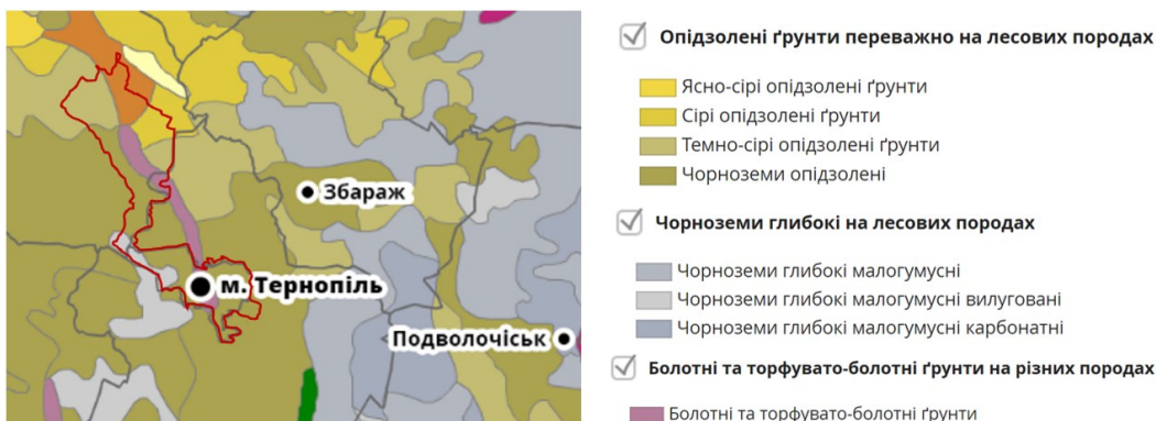
Рис. 3.1.1. Карта ґрунтів на території Тернопільської міської територіальної громади 5
