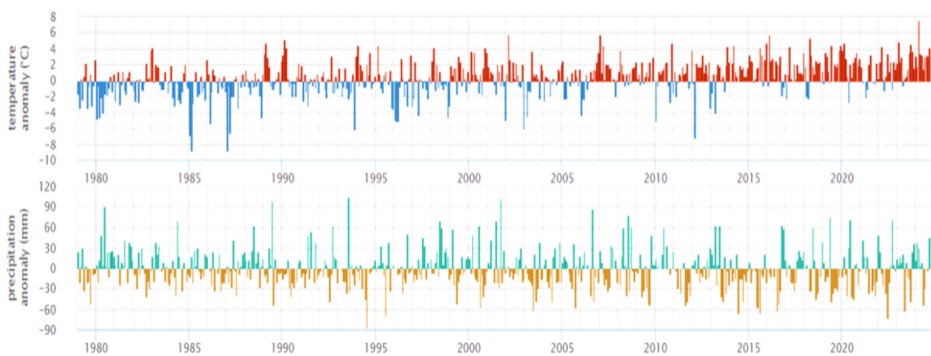
Рис. 3.1.3. Історичні дані клімату і погоди у Тернопільській міській територіальній громаді за тридцятиріччя (1979-2024 роки) 14
